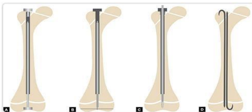
а) Dubow–Bailey таяқшасы; в) Cho бекітілетін таяқша; с) Fassier–Duval телескопиялық жүйесі; d) Rush таяқшалары [112].
